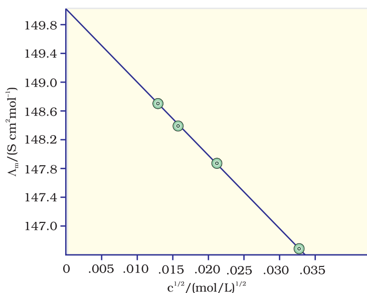
चित्र 3.7- c^{1/2} के विरुद्ध \dot{\Lambda}_m में परिवर्तन
