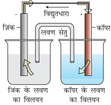
चित्र 3.1- डैन्यल सेल जिसमें जिंक एवं कॉपर इलेक्ट्रोड अपने-अपने लवणों के विलयनों में निमज्ज हैं।
