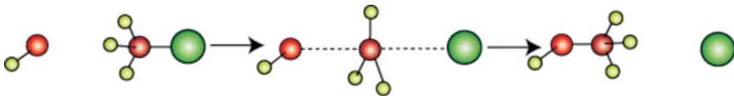
चित्र 10.2— लाल बिंदु आक्रमणकारी हाइड्रॉक्साइड आयन को तथा हरा बिंदु निकलने वाले हैलाइड आयन को प्रदर्शित करता है।
